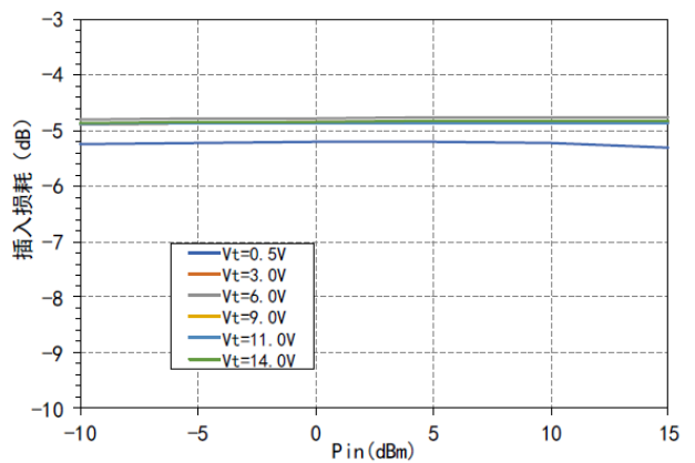
插入损耗VS Pin@1.5GHz
