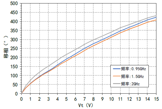
移相VS Vt@Pin=-10dBm
