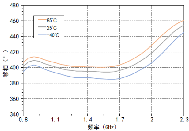
移相VS频率@Vt=14V
